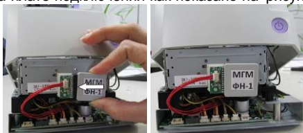
Рисунок 7 – Порядок установки фискального накопителя
